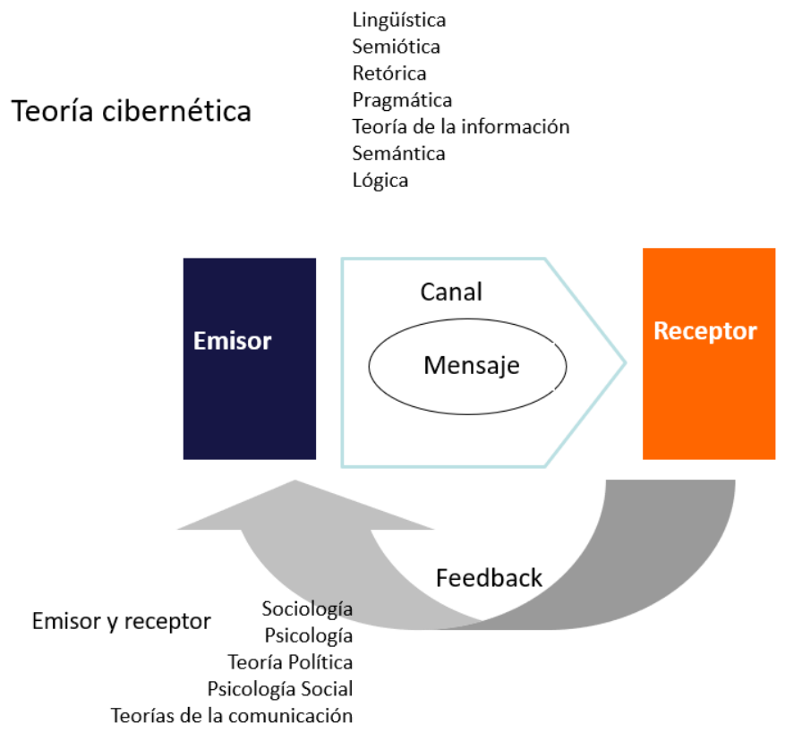
Figura 1 – teoría cibernética
