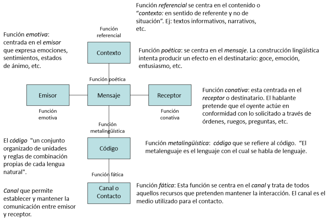
Figura 2 – Teoría lingüística
