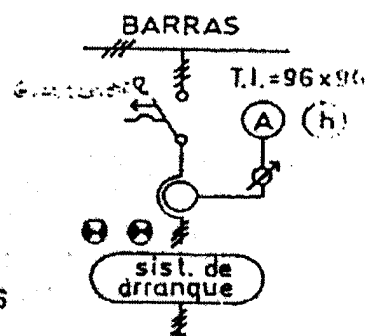
c) Salida de circuito para motor
