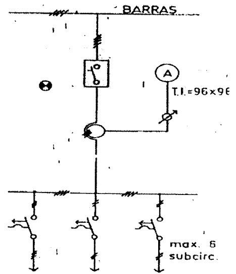
e) Salida a tableros subseccionales
