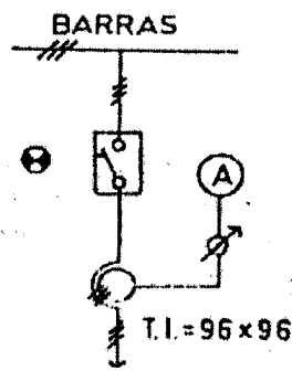
b) Salida a circuito fuerza
