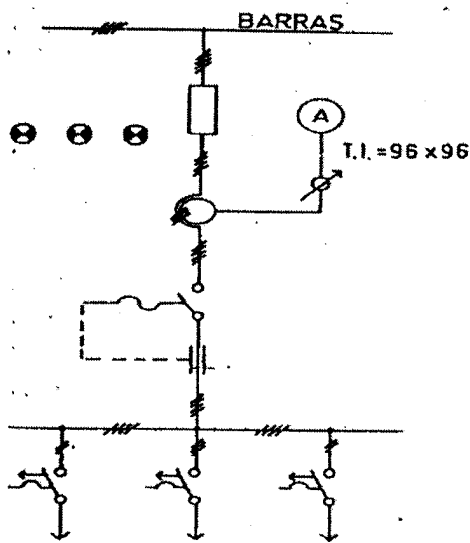
d) Salidas para iluminación y tomas
